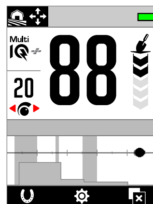
Todos os metais desativado — O Padrão de discriminação está ativo.
